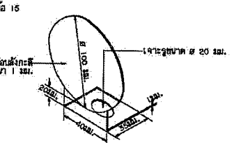
แบบติดตั้งเครื่องหมายทาง
