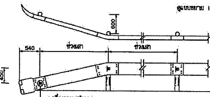
แบบขยาย 1. แสดงการติดตั้งและหน่วยขยาย GUARD RAIL
