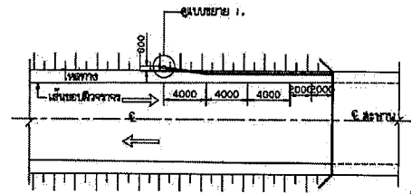
แบบติดตั้ง GUARD RAIL PRESERVE
