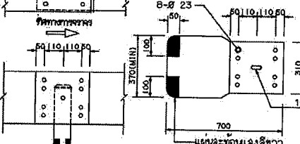
แบบติดตั้งเครื่องหมายทาง
