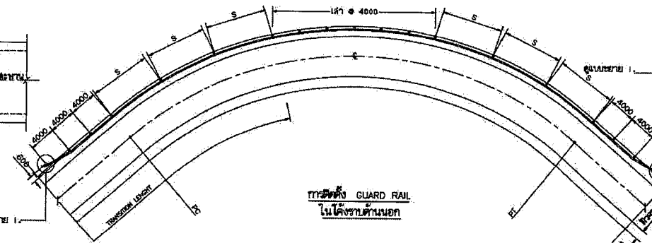
แบบติดตั้ง GUARD RAIL PRESERVE
