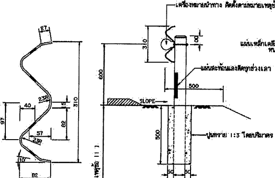
รูปตัด GUARD RAIL
