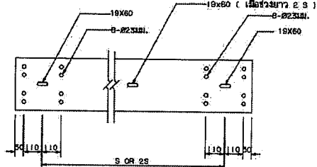
แบบติดตั้ง GUARD RAIL ในโค้งขนาบด้านนอก
